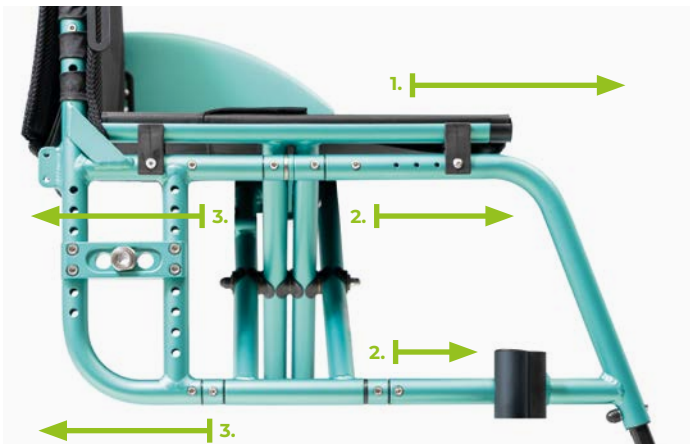
Profondità telaio allungabile in avanti (2) o indietro (3). Adjustable frame, forwards (2) or backwards (3).
