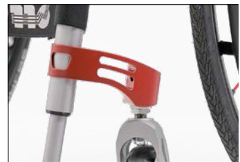
Piastra EAR colorata e regolabile in altezza e inclinazione. Colourful EAR plate: adjustable in height and angle.
