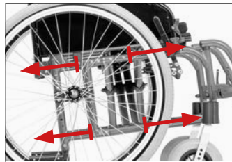
Profondità telaio allungabile in avanti (2) o indietro (3). Adjustable frame, forwards (2) or backwards (3).
